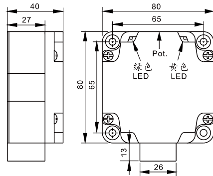
尺寸图(单位:mm)
